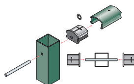
Tarpinio stulpo jungtis
